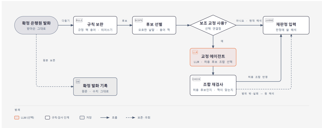
도식 4. 규칙 기반 용어 보완과 선택적인 LLM 보조 교정의 경계.
